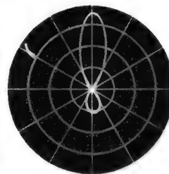
Bild 10. Richtcharakteristik der 9-Element-Antenne für den Kanal 9 = 189 MHz. Der Gewinn ist größer als in Bild 7
