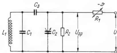
Bild 5. Schaltung zur Erzielung eines negativen Temperaturbeiwertes der Sperrschichtkapazität C_2
