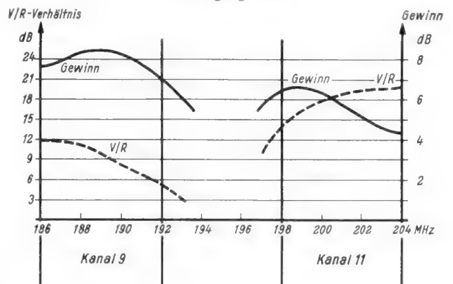
Bild 12. Gewinn und V/R-Verhältnis der 9-Element-Janus-Antenne
