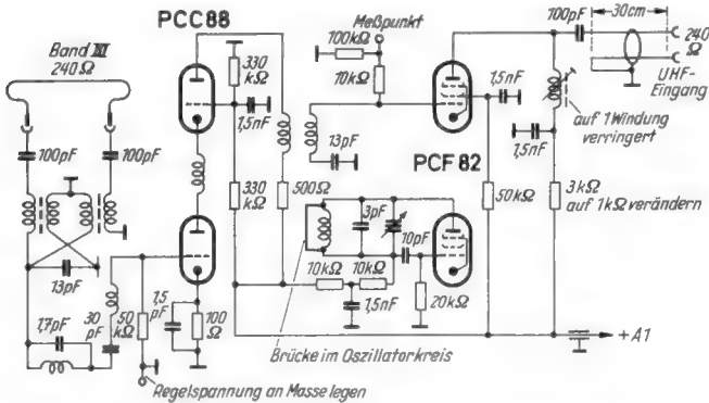
Bild 1. Umbau eines VHF-Tuners in einen UHF-Konverter
