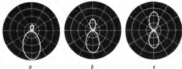
Bild 3. Umkippen der Richtwirkung bei einer 2-Element-Janus-Antenne für f_0 = 60 MHz
