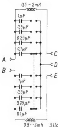
Bild 1. Schaltung des Experimentierfilters
