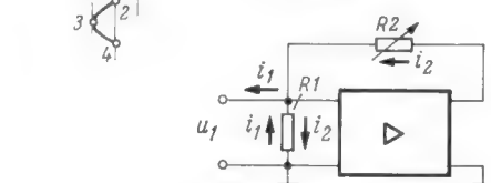
Bild 2. Aussteuerung des negativen Kennlinienteiles durch eine Wechselspannung
