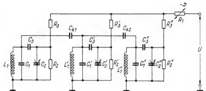
Bild 7. Temperaturkompensiertes Dreikreis-Filter
