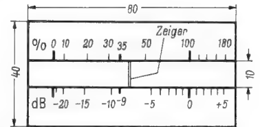
Bild 1. Ungefährer Skalenverlauf. Die Maße geben die Größe des Papierskalenblattes an. Genaue Angaben sind infolge der Toleranzen der Bauteile nicht möglich
