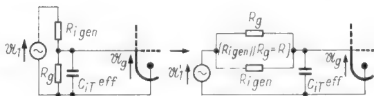
Bild 2. Prinzipschaltung (a) und Ersatzschaltung (b) zur Ermittlung der oberen Grenzfrequenz eines Verstärkereinganges
