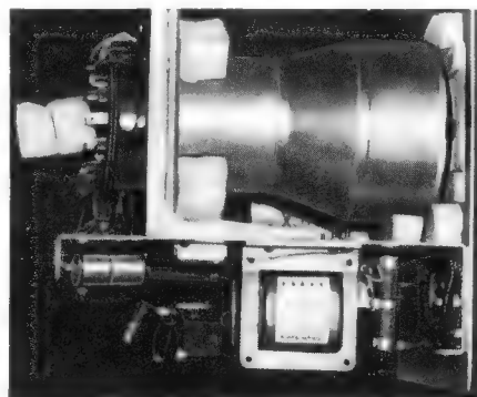
Bild 5. Einbau der Elektronenstrahlröhre
