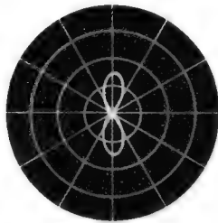
Bild 6. Richtcharakteristik zwischen Kanal 9 und 11, entsprechend einer Frequenz von 195 MHz
