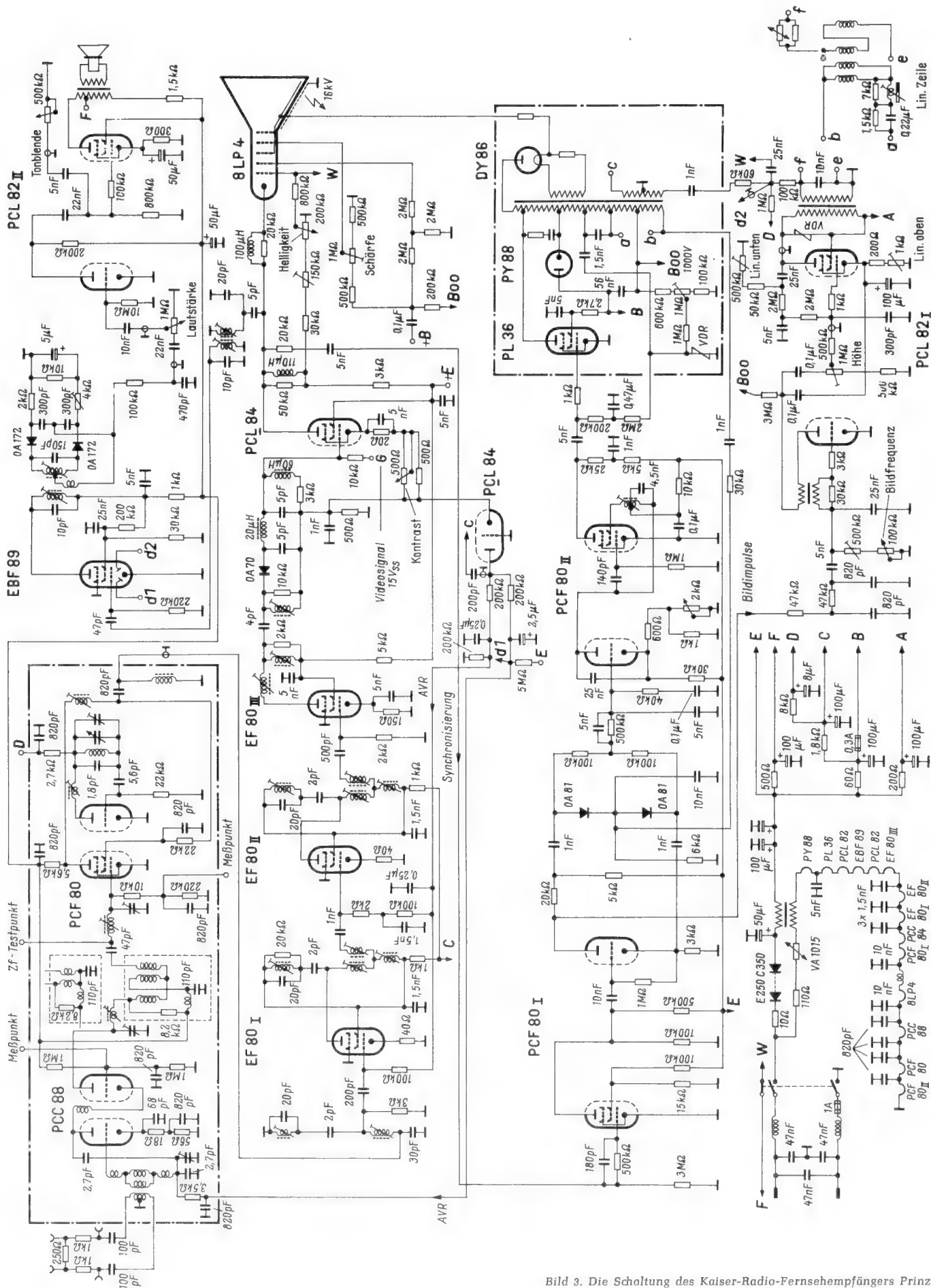
Bild 3. Die Schaltung des Kaiser-Radio-Fernsehempfängers Prinz
