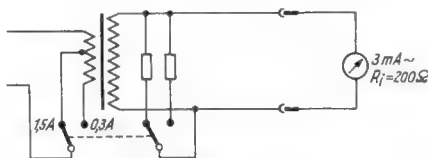
Bild 3. Stromwandler für zwei Meßbereiche mit Abgleichwiderständen zum Anschluß an ein Vielfach-Meßgerät
