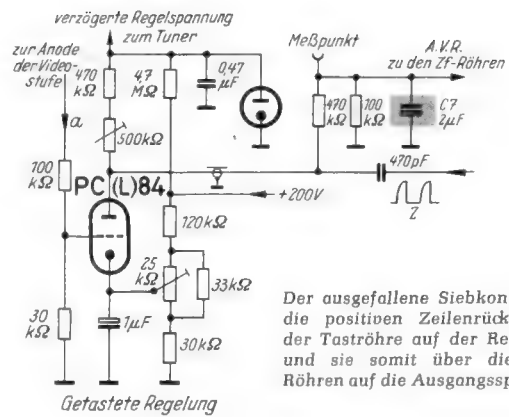
Gefastete Regelung
