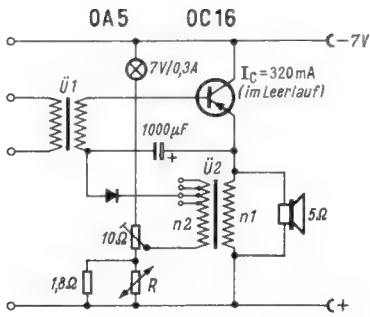
Bild 13. 4-W-Endstufe mit gleitendem Arbeitspunkt
