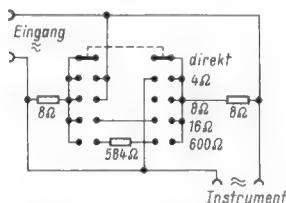
Bild 2. Schaltung eines Zusatzgerätes für Tonfrequenz-Leistungsmessungen (Outputmeter)
