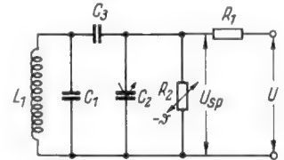
Bild 4. Schaltung zur Erzielung eines positiven Temperaturbeiwertes der Sperrschichtkapazität C 2
