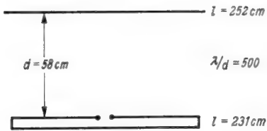
Bild 4. Abmessungen der Versuchsentenne mit zwei Elementen
