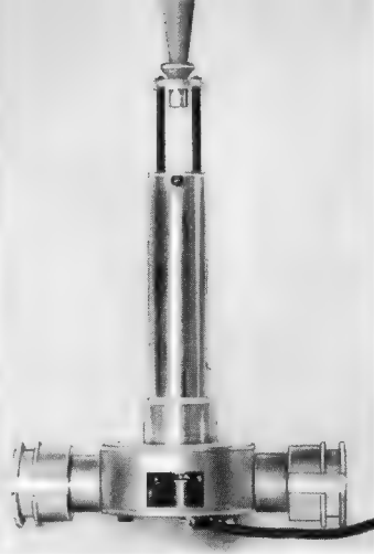
Bild 8. Mechanischer Aufbau der Schaltung Bild 7
