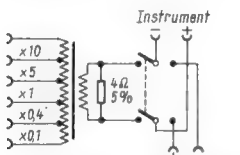
Bild 1. Schaltung eines Meßwandlers zur Unterteilung der vorhandenen Wechselstrommeßbereiche
