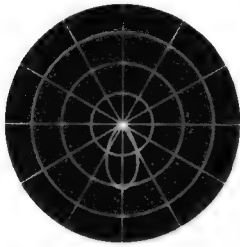
Bild 5. Richtkeule der 5-Element-Yagi-Antenne für die Mitte von Kanal 11 = 201 MHz
