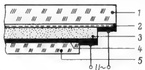
Bild 1. Prinzip der Elektro-Lumineszenz-Platte; 1 = Deckplatte, 2 = durchsichtige Elektrodenschicht mit Anschlußstreifen, 3 = Dielektrikum mit Leuchtstoff-Kristallen, 4 = Elektrodenschicht mit Anschlußstreifen, 5 = Trägerplatte
