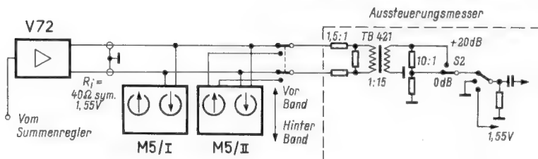
Bild 9. Schaltung mit symmetrischem Eingang für Verwendung mit reinen Studiogeräten
