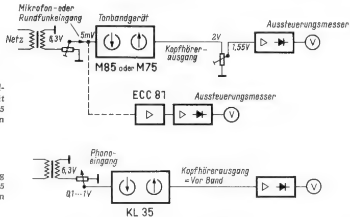
Bild 9. Schaltung mit symmetrischem Eingang für Verwendung mit reinen Studiogeräten
