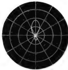
Bild 7. Richtkeule der 5-Element-Janus-Antenne für die Mitte von Kanal 9 = 189 MHz
