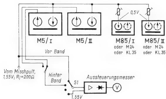
Bild 8. Blockschaltbild der Anlage, für die das Gerät entwickelt wurde
