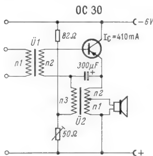
Bild 10. 1-W-Endstufe für A-Betrieb
