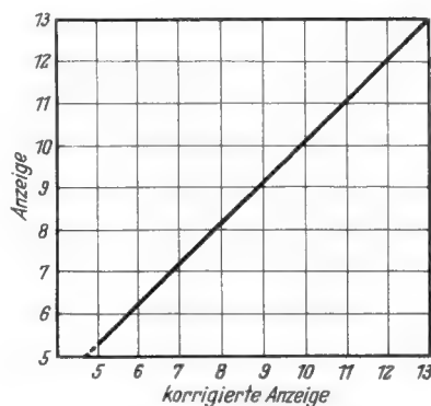
Bild 1. Skalendifferenz im Anfangsbereich der Wechselstromskala eines Vielfach-Meßgerätes
