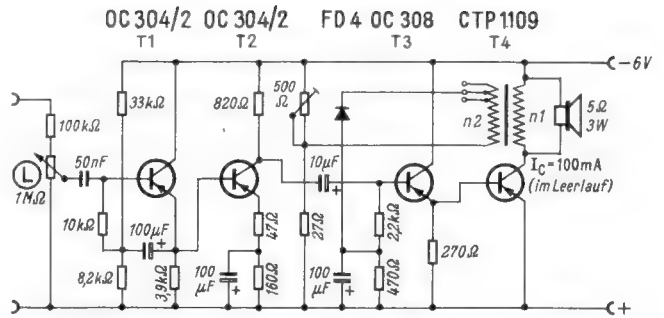
Bild 13. 4-W-Endstufe mit gleitendem Arbeitspunkt
