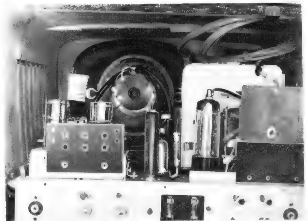
Bild 2. Blick in das Innere des Gerätes; trotz der geringen äußeren Abmessungen ist über den Röhren des Horizontalchassis noch reichlich Raum vorhanden
