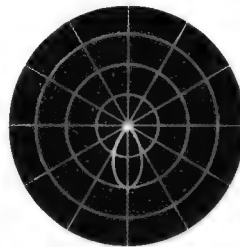
Bild 9. Richtcharakteristik der 9-Element-Janus-Antenne für Kanal 11 = 201 MHz
