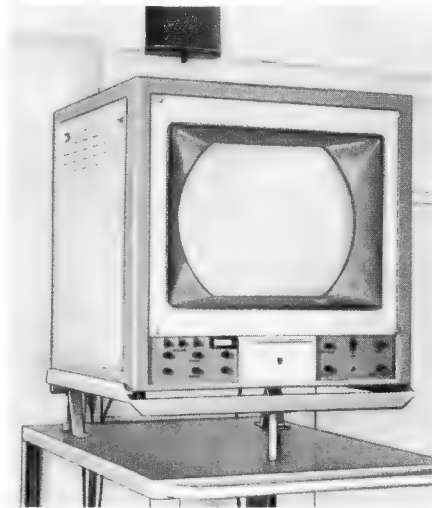
Bild 2. 53-cm-Farbfernseh-Monitor im Leichtmetallgehäuse mit Shadow-Mask-Bildröhre (Eingang: Videosignal + 1,4 V_{SS} an 75 \Omega )
