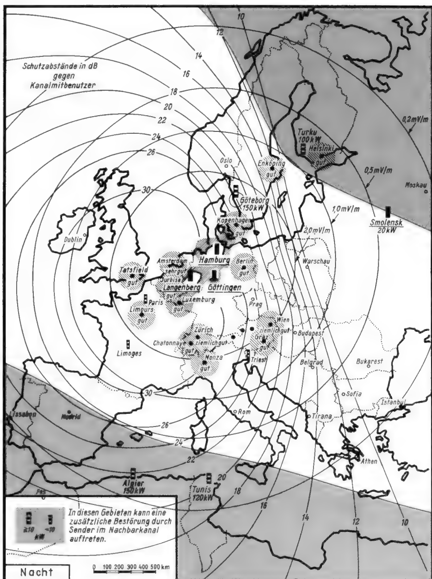
Bild 2. Nachthörbarkeit der Frequenz 971 kHz (Hamburg/Langenberg/Göttingen). Diese Karte wurde in Wittsmoor unter Mithilfe zahlreicher ausländischer Meßstellen gezeichnet. Kanalmitbenutzer: Smolensk/UdSSR
