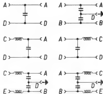
Bild 2. Sechs mit dem Experimentierfilter herstellbare Anordnungen
