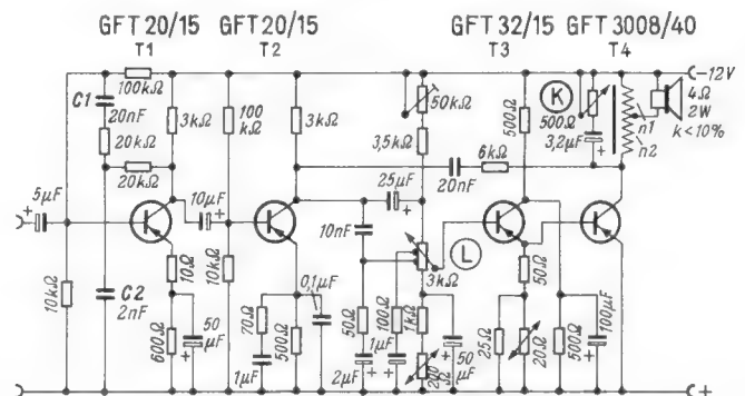
Bild 12. Tonfrequenzverstärker mit Höhen- und Tiefenanhebung sowie 2-W-Eintakt-Endstufe
