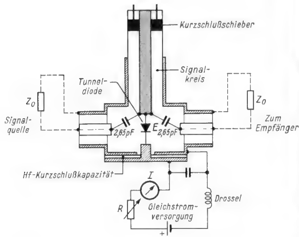
Bild 7. Praktischer Aufbau der Schaltung nach Bild 6 für f = 400 \dots 800 MHz mit einer Telefonkenn-Versuchs-Tunnel-Diode, Muster Nr. 37
