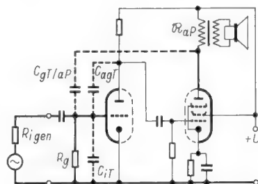
Bild 1. Prinzipschaltung eines zweistufigen Verstärkers. Die den Rückkopplungsgrad Anode-Pentode/Gitter-Triode und die obere Grenzfrequenz des Verstärkereinganges bestimmenden Schaltungsglieder sind stark ausgezogen
