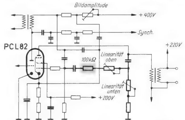
Die Gegenkopplung in der Bildkipp-Endstufe beeinflusst die Bildhöhe und Bildlinearität
