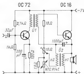
Bild 11. 4-W-Endstufe für A-Betrieb
