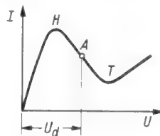
Bild 1. Grundsätzliche Kennlinie einer Esaki-Diode
