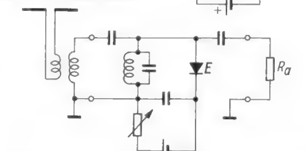
Bild 6. Erweiterung der Schaltung Bild 5 zu einer Vierpolstufe
