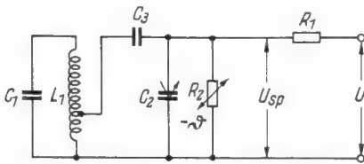
Bild 6. Schaltung zur Erzielung einer größeren Kreisgüte
